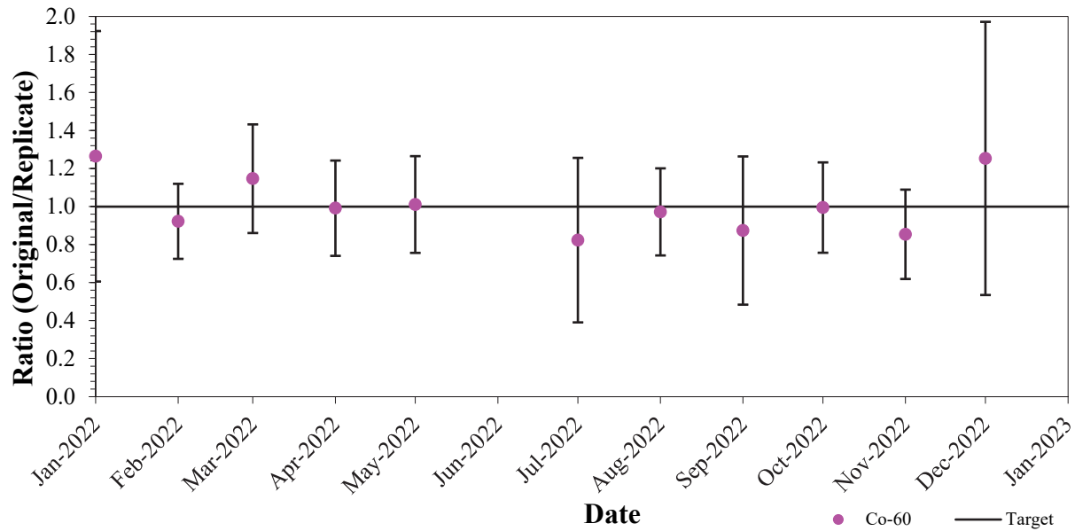
Image 7.05 : Performance du cobalt-60 (AQ interne – double/multiple) (couleur)
