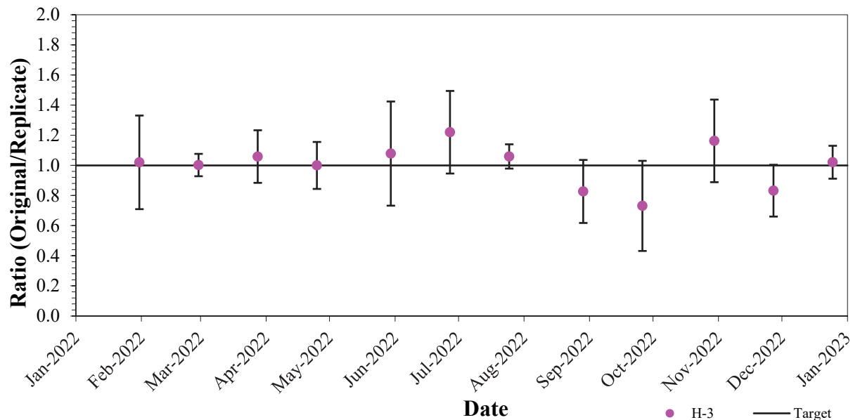
Image 7.06 : Performance du tritium (AQ interne – Double/multiple) (couleur)
