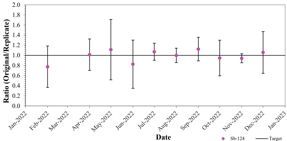
Image 7.12 : Performance du Sb-124 (AQ interne – double/multiple) (couleur)
