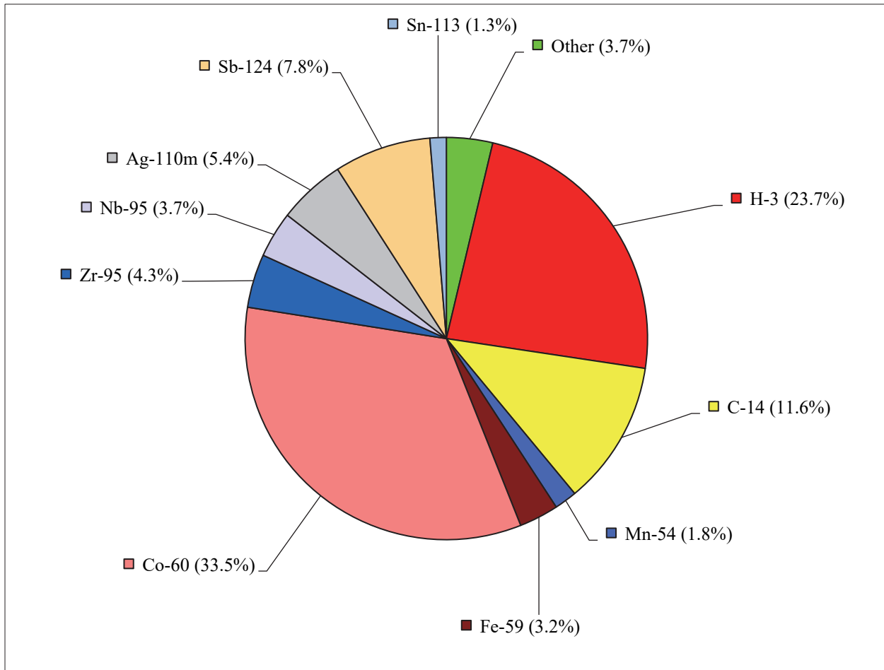
Image 6.02 : Contribution des radionucléides à la dose totale (dans les liquides) – 2022 (couleur)
