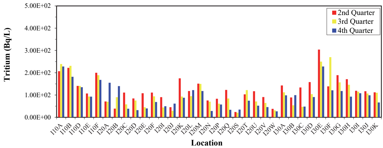
Image 4.20 : Tritium (eau de trou de forage, IGDRS) 2022 (couleur)
