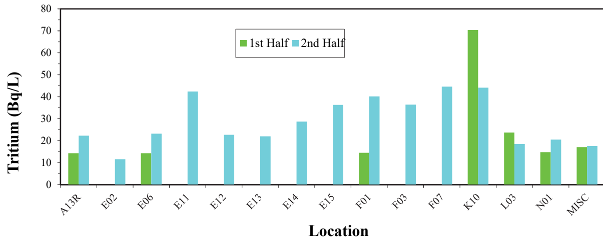
Image 4.11 : Tritium (eau de puits) 2022 (couleur)
