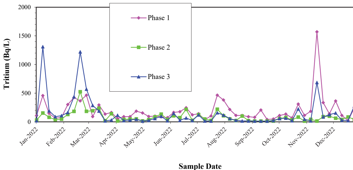
Image 4.21 : Tritium (eau du canal Parshall, IGDRS) 2022 (couleur)
