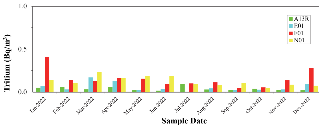
Image 4.03 : Tritium (vapeur d'eau) aux postes éloignés de mesure de la qualité de l'air (couleur)
