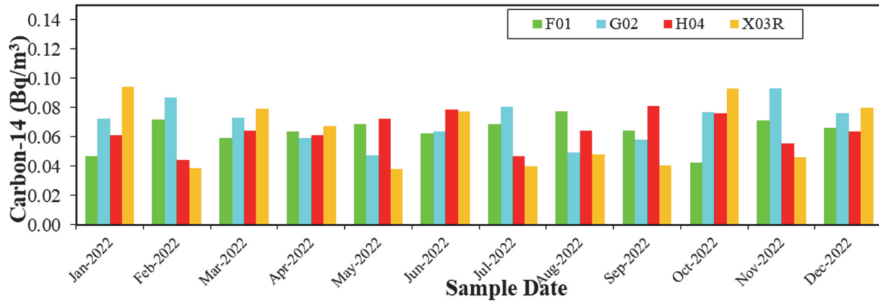
Image 4.07 : Carbone-14 (dioxyde de carbone) (couleur)
