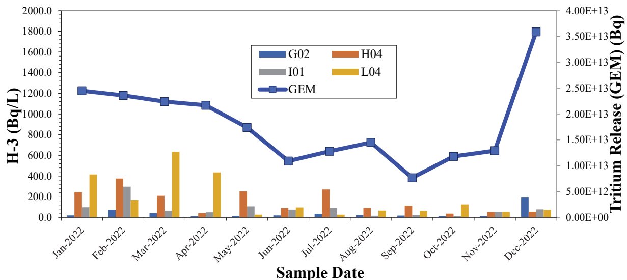
Image 4.14 : Résultats relatifs aux émissions de H-3 gazeux et de tritium (précipitations) (couleur)
