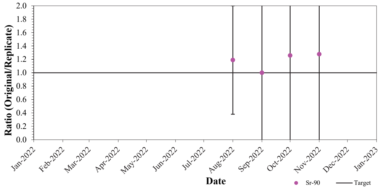
Image 7.09 : Performance du strontium-90 (AQ interne – Double/multiple) (couleur)
