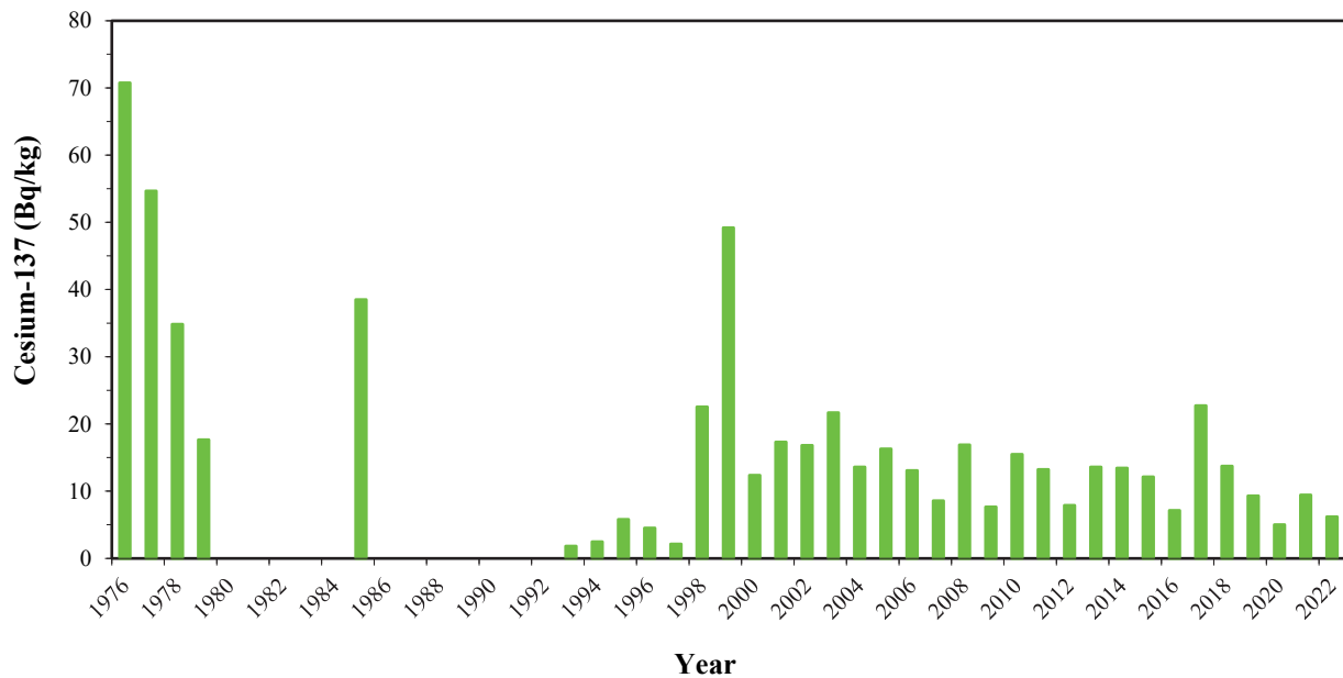
Image 5.05 : Césium-137 (terre) (couleur)
