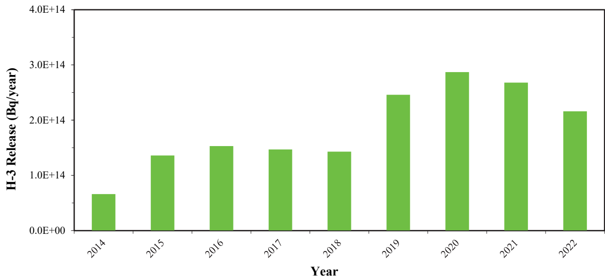
Image 5.02 : Émissions atmosphériques de H-3 (couleur)
