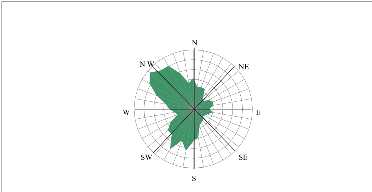
Image 4.22 : Rose des vents de Point Lepreau (2022) (couleur)
