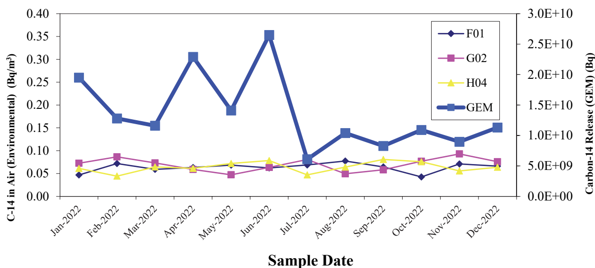
Image 4.09 : Résultats relatifs aux émissions de C-14 gazeux et de C-14 (vapeur d'eau) (couleur)
