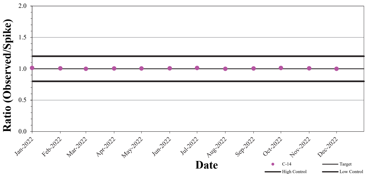
Image 7.15 : Performance du C-14 (AQ interne – pics) (couleur)
