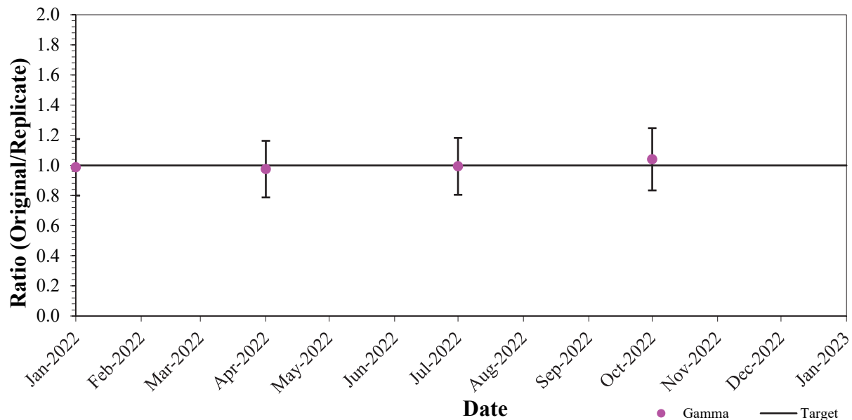
Image 7.08 : Performance du rayonnement gamma (AQ interne – Double/multiple) (couleur)
