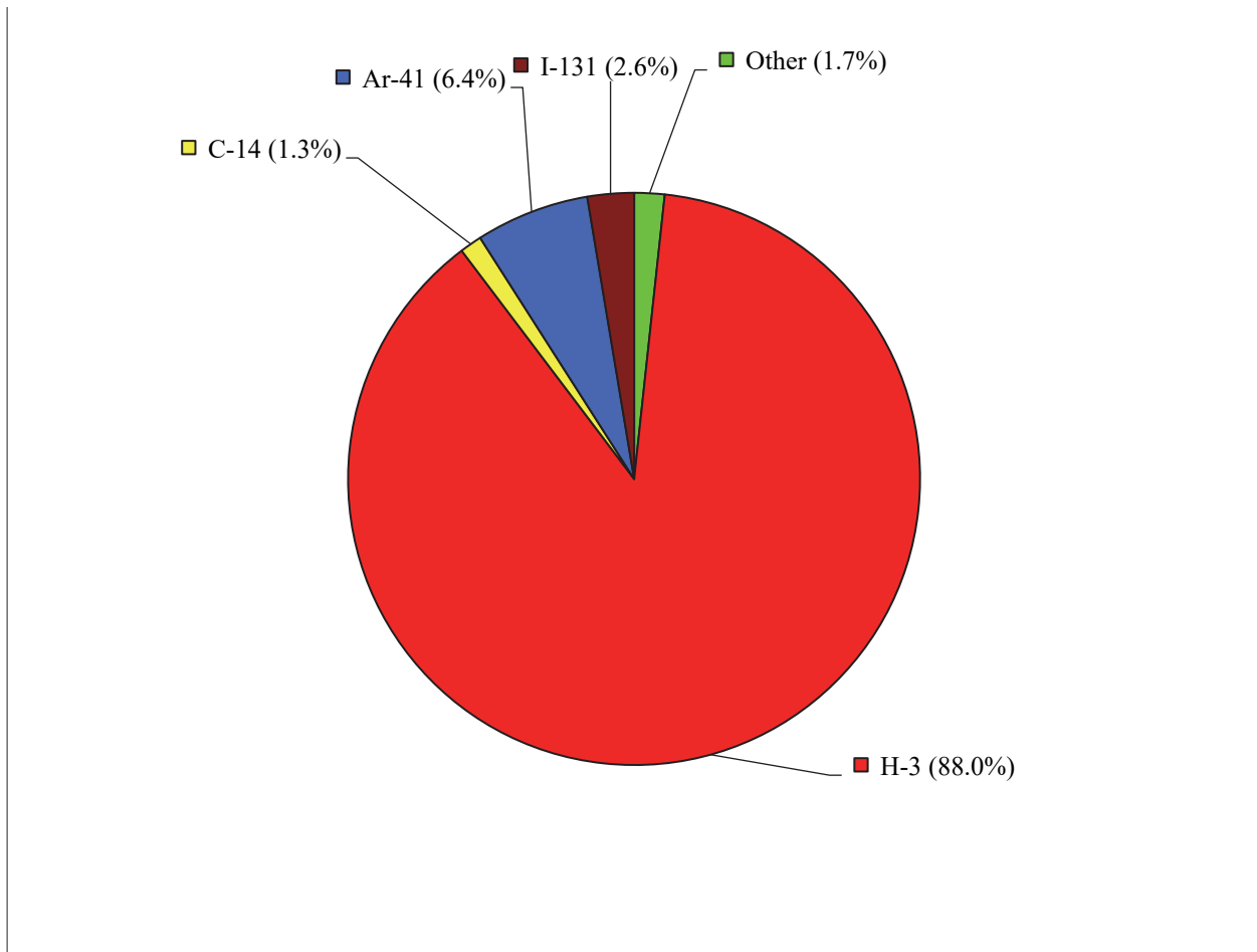
Image 6.01 : Contribution des radionucléides à la dose totale (dans l'air) – 2022 (couleur)
