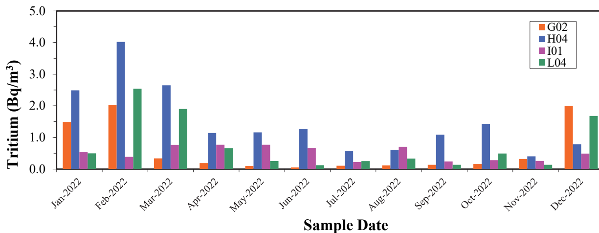
Image 4.04 : Tritium (vapeur d'eau) aux postes rapprochés de mesure de la qualité de l'air (couleur)
