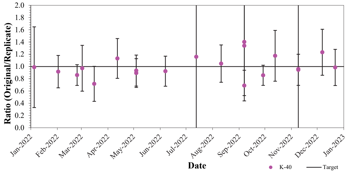
Image 7.07 : Performance du potassium-40 (AQ interne – Double/multiple) (couleur)
