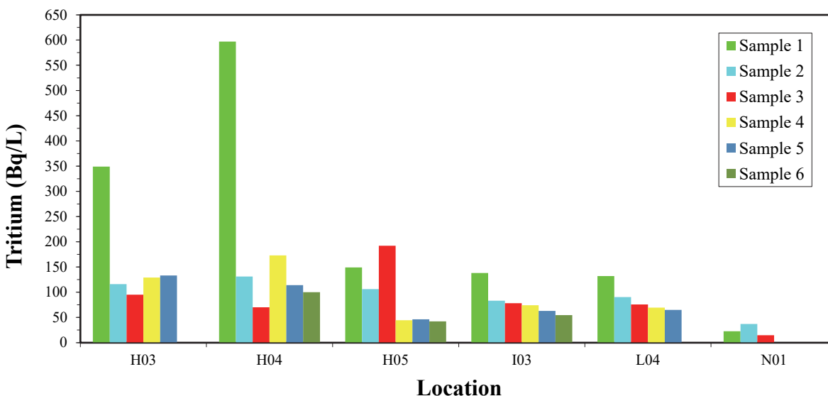
Image 4.12 : Tritium (étangs, flaques d'eau et eau de surface) 2022 (couleur)
