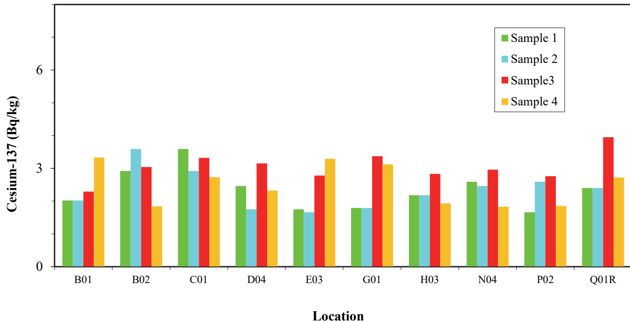
Image 4.18 : Césium-137 (sédiments) 2022 (couleur)
