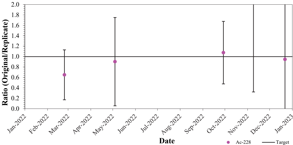
Image 7.13 : Performance de l'actinium-228 (AQ interne – double/multiple) (couleur)
