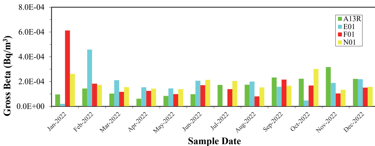
Image 4.01 : Radioactivité bêta brute (particules dans l'air) aux postes éloignés de mesure de la qualité de l'air (couleur)
