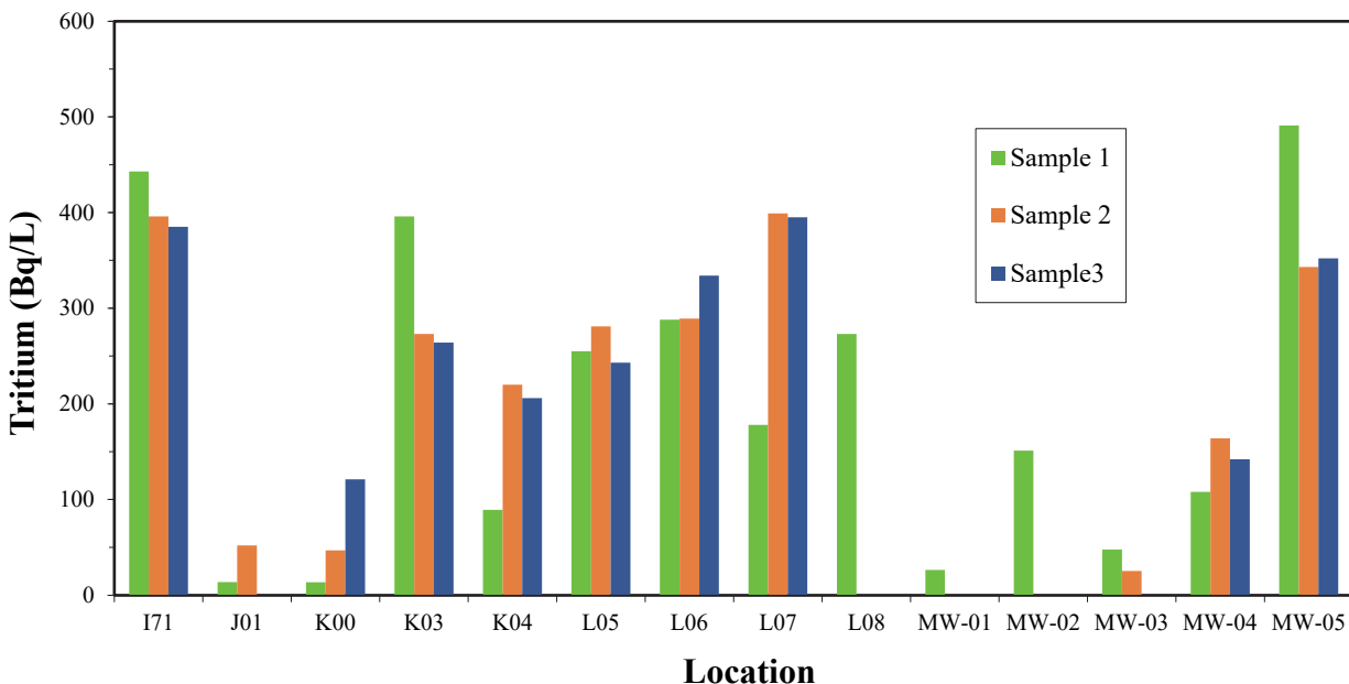
Image 4.15 : Tritium (Surveillance de l'eau de puits près de la centrale) 2022 (couleur)
