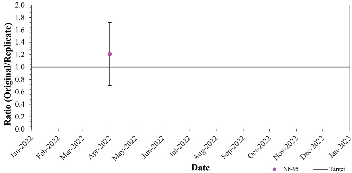
Image 7.11 : Performance du niobium-95 (AQ interne – Double/multiple) (couleur)
