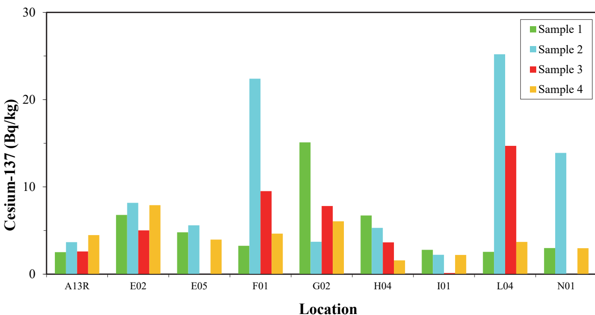
Image 4.13 : Césium-137 (terre) 2022 (couleur)
