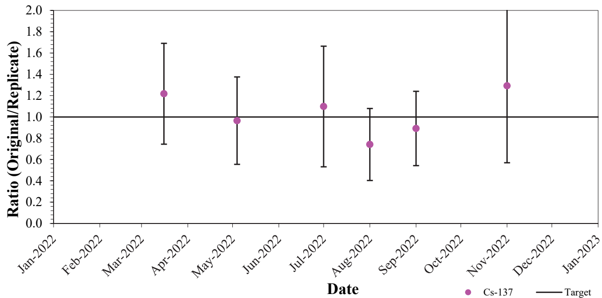
Image 7.10 : Performance du Cs-137 (AQ interne - Double/multiple) (couleur)
